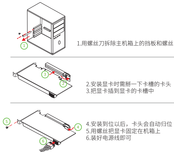
图2 -10 显卡安装
