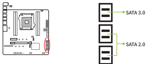
图2 -11 SATA接口
