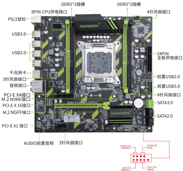
图1-1 X79-ZD3 主板图解
